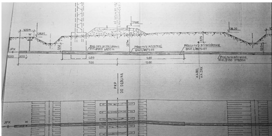
Fragment dokumentacji na potrzeby przeprowadzenia gazociągu pod torami linii kolejowej relacji Warszawa - Dęblin - Fot. dokumentu udostępnionego przez Janusza Górskiego
